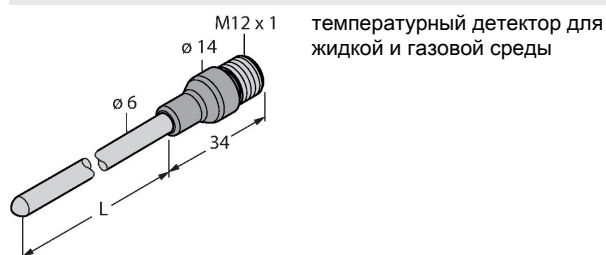
TP-306A-CF-H1141-L1000 9910479
