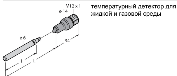
TP-306A-CF-H1141-L1000 9910479
